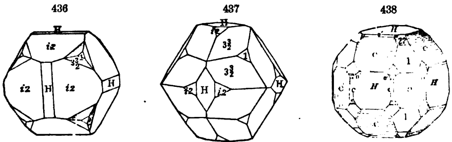
Rossie.
